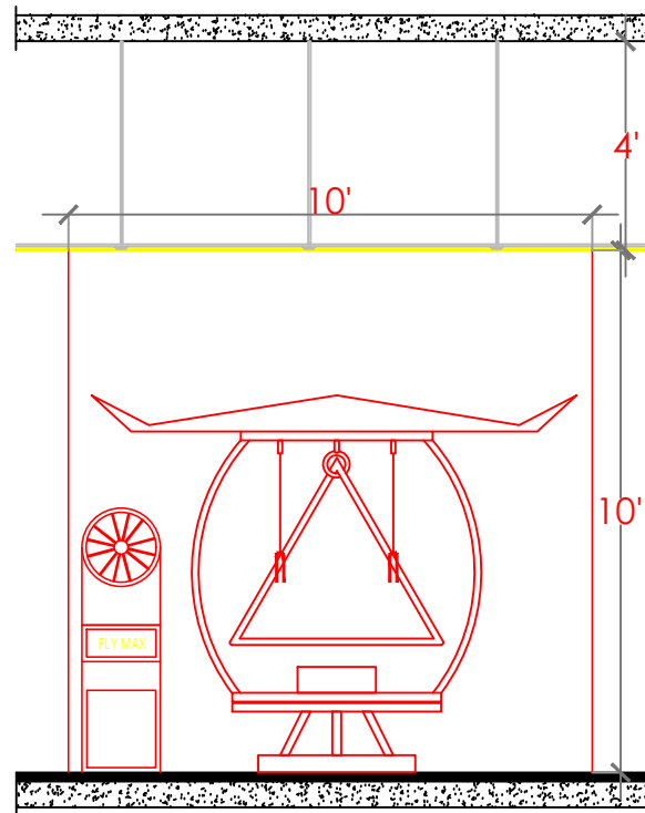
SECTION - C1
