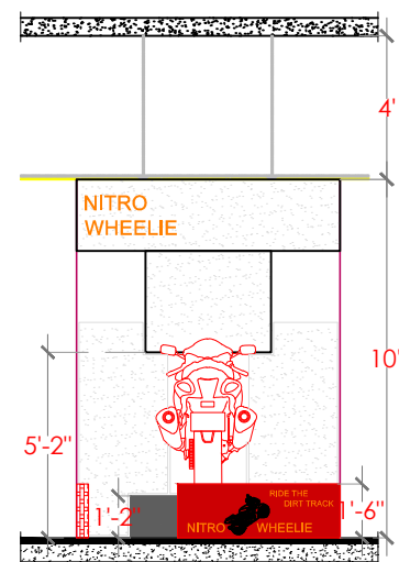
SECTION - I2
