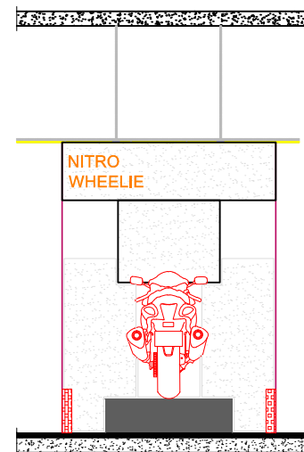
SECTION - I1
